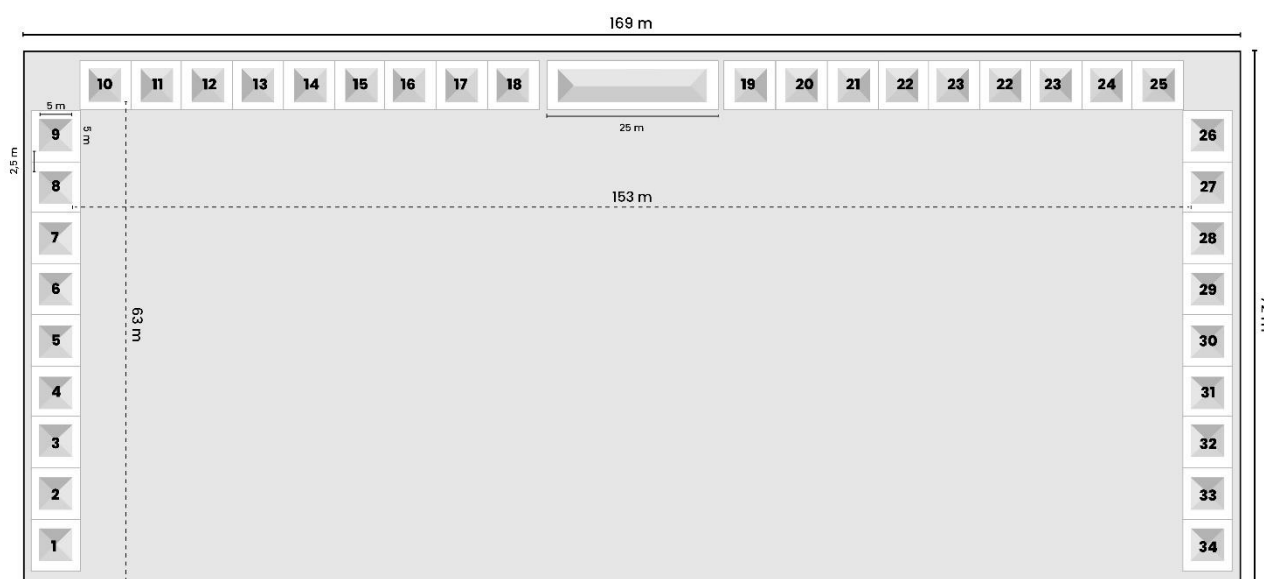
DENAH LAPANGAN UTAMA BUPERTA CIBUBUR
